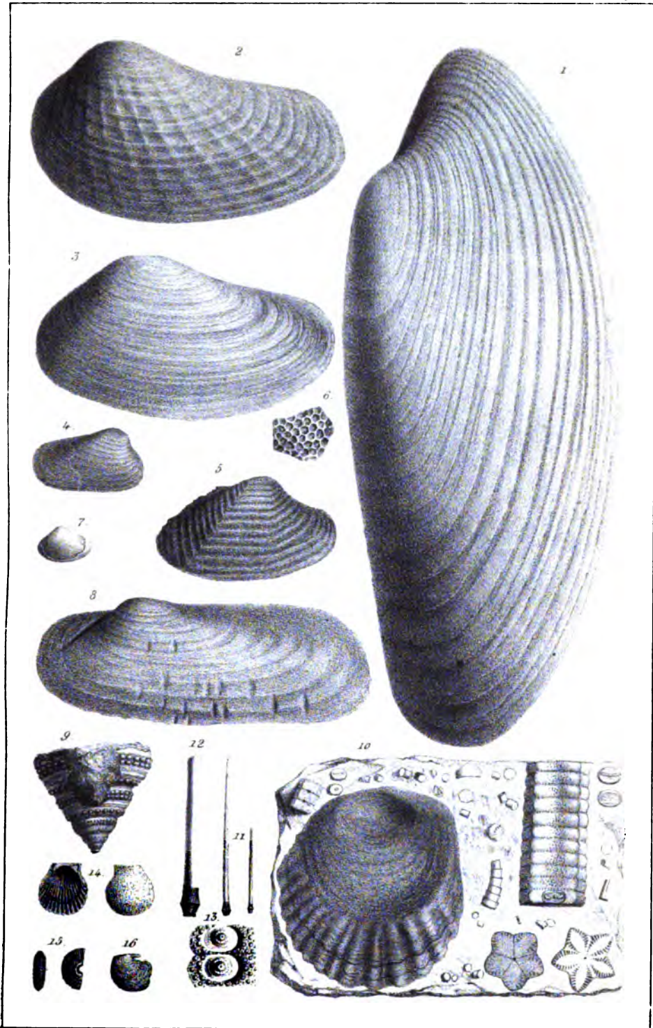
Quenstedt, Jurat.
